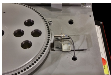
Fine corsa
